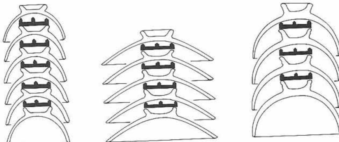
Σχεδιαστική απεικόνιση του στοιβάγματος των εφυαλωμένων αγγείων στο καμίνι μέσω τριποδίσκων.
