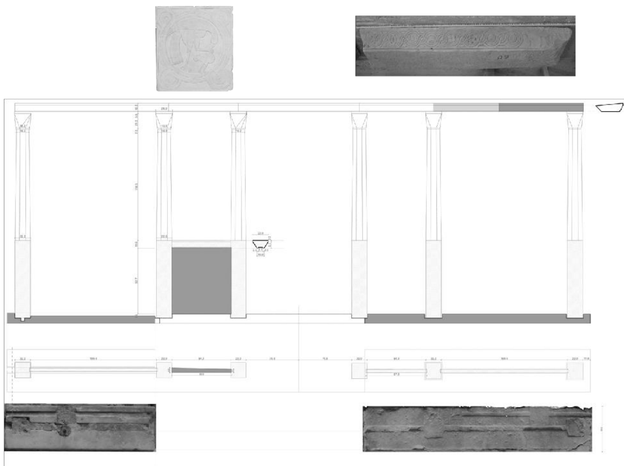
εικ. 3: Αφαιρετική σχεδιαστική αποκατάσταση μεσοβυζαντινού τέμπλου. Τμήματα στυλοβάτη, τμήμα επιστυλίου και θωράκιο (σχεδίαση Μ. Χατζημιχάλη).
